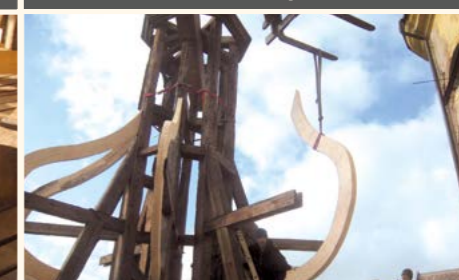
Montáž ramenátů do konstrukce krovu věže
